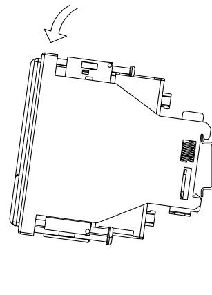
Rys.3 Zakładanie zestawu na szynę TS35.
